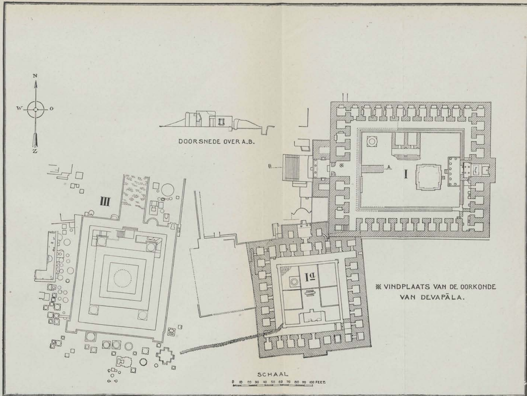
Pl. III. Plattegrond van de te Nālandā ontgraven bouwwerken. (Naar de teekeningen van Hirananda Shastri in ASR — EC 1919—20 en ASR — CC 1920—21).
