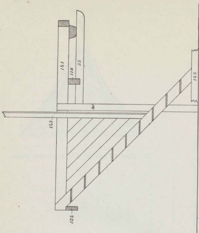
15. Trap (zij-aanzicht).
