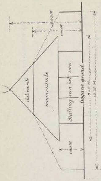
11. Schematische breedte-doorsnede der Rotneese woning.
