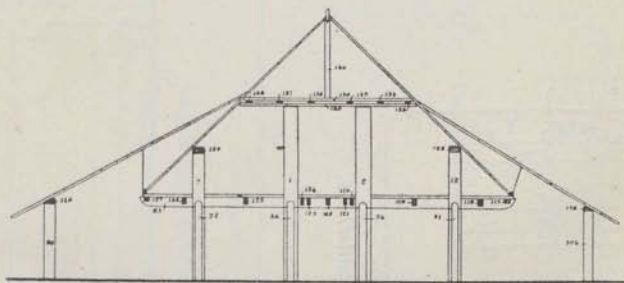
2. Breedte-doorsnede van het huis.
