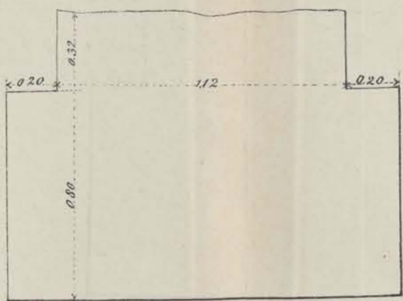
Fig. 5 Fundering van den ringmuur
